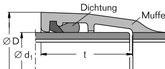
Muffe für Rohre, DN 700 bis DN 1000 Langmuffen Fabrikat Buderus
